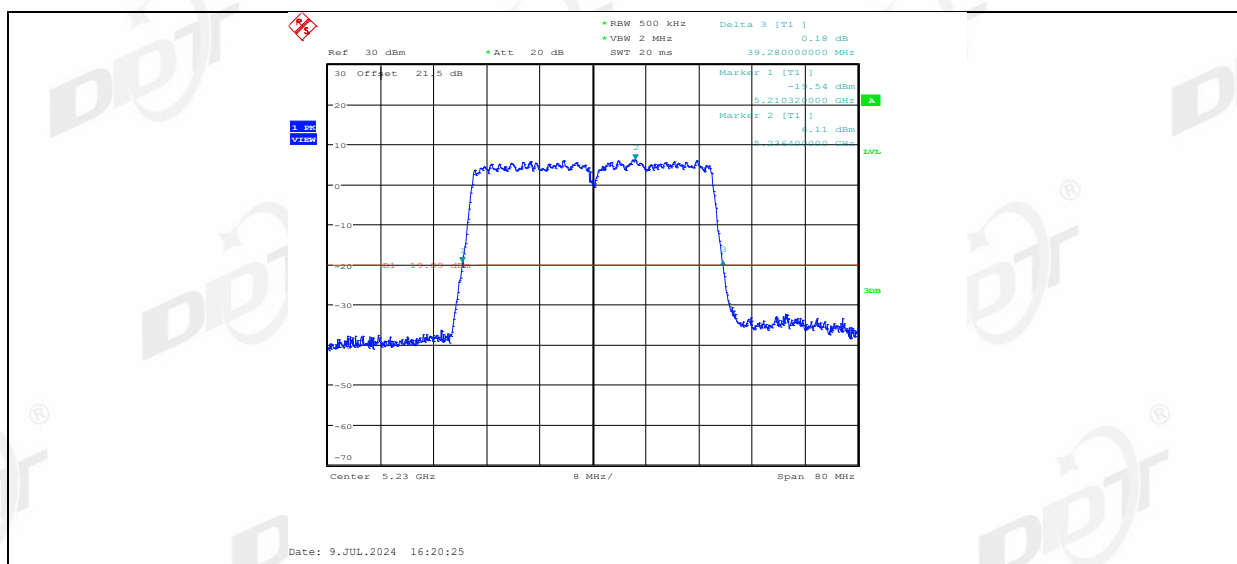
11AX40MIMO Ant1 5270
