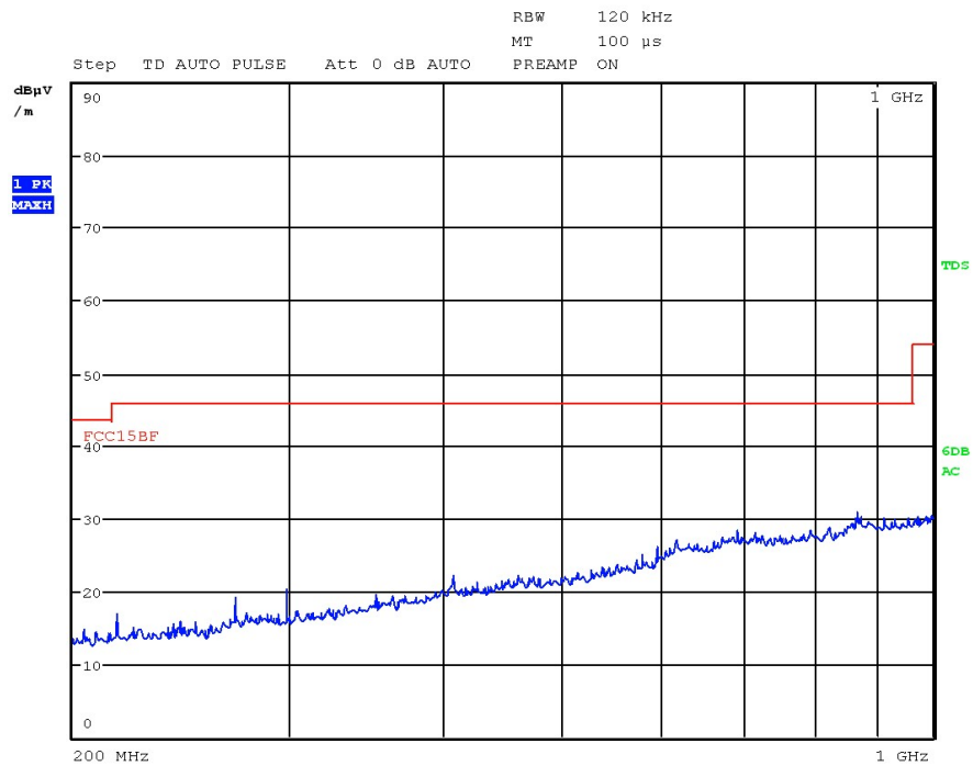
200MHz~1000MHz Vertical
