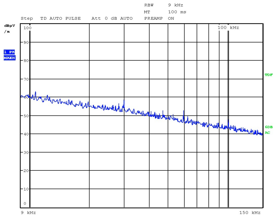
9kHz~150kHz Face
