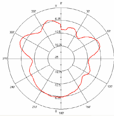
2.4 GHz H-Plane Vertical
