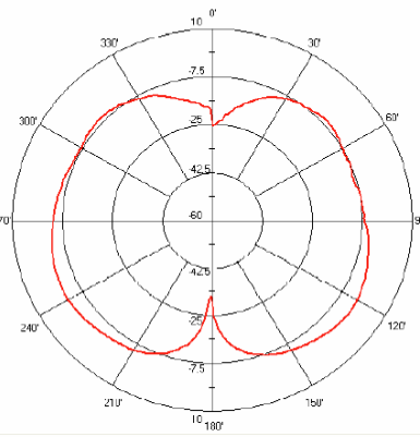
2.4 GHz H-Plane Horizontal
