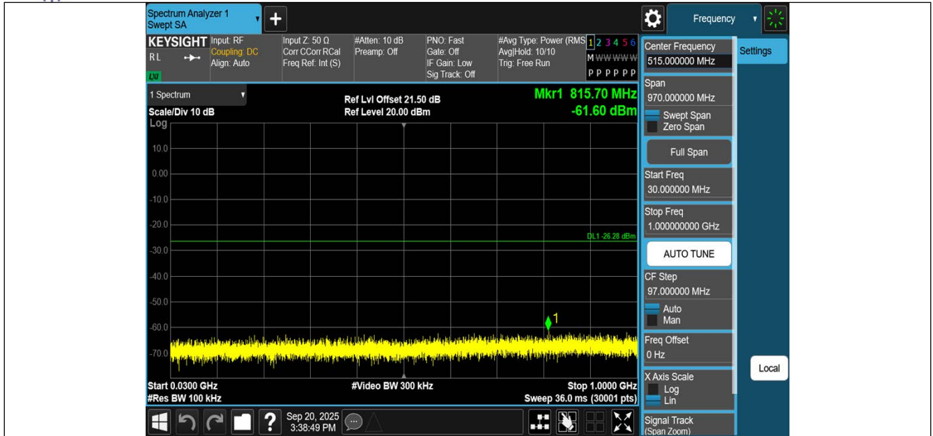
11G-Ant1-2412-30~1000-PASS
