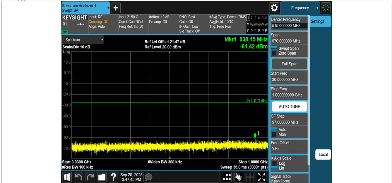
11G-Ant1-2462-30~1000-PASS
