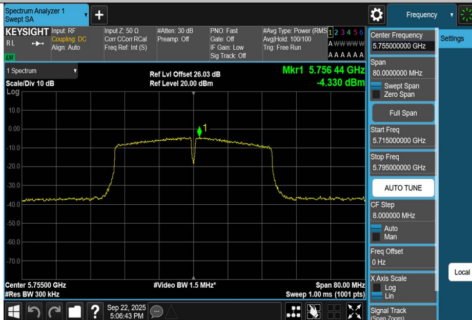
11N40SISO-Ant1-5755-PASS
