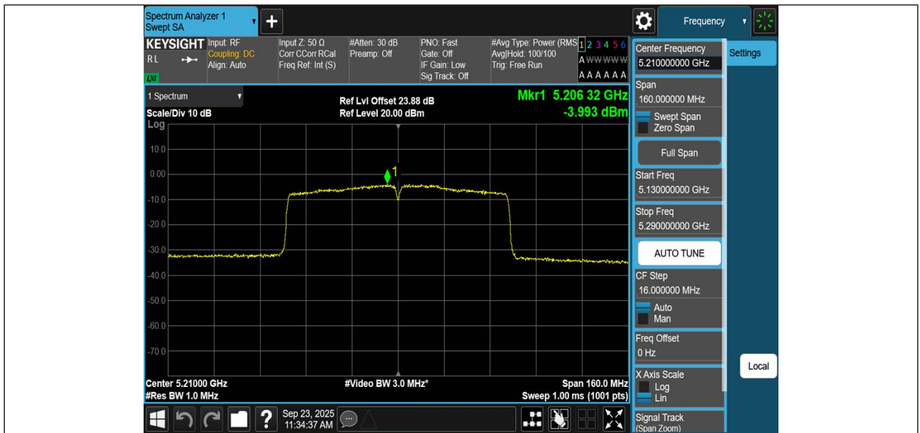
11AC80SISO-Ant1-5210-PASS
