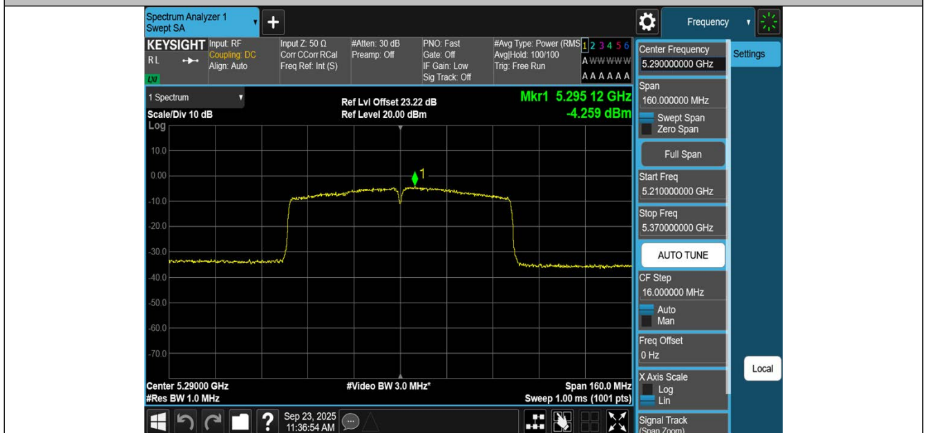
11AC80SISO-Ant1-5290-PASS
