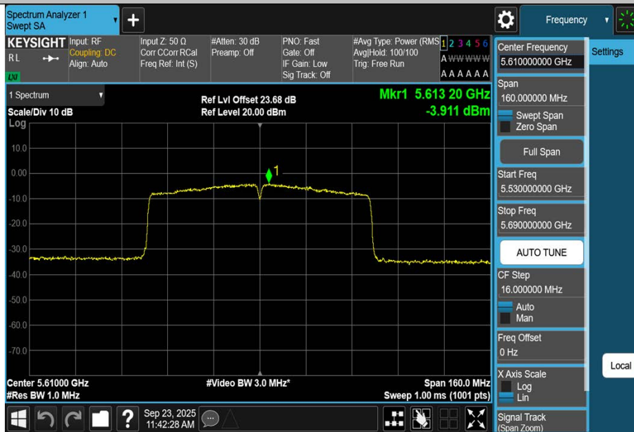
11AC80SISO-Ant1-5610-PASS
