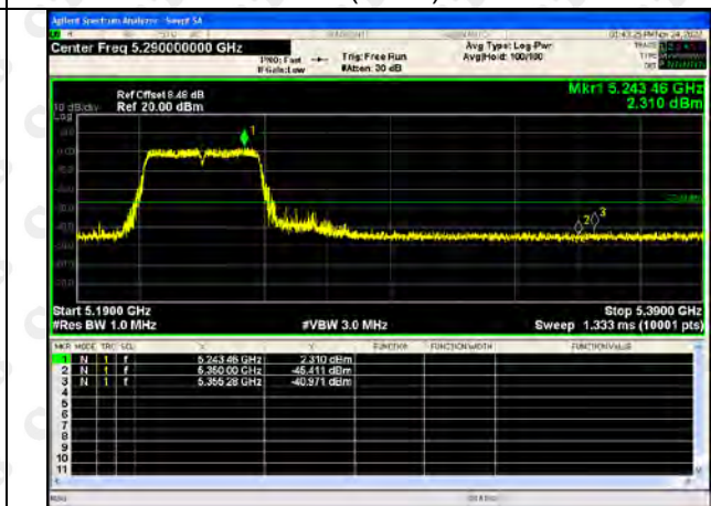
802.11n(HT40)-5230
