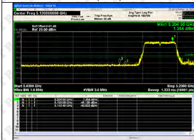
802.11ac(VH80)-5210
