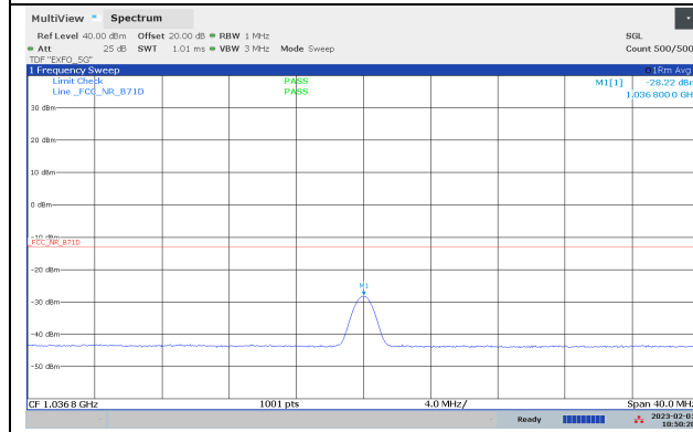
Ch126800 BW10 1036.8MHz
