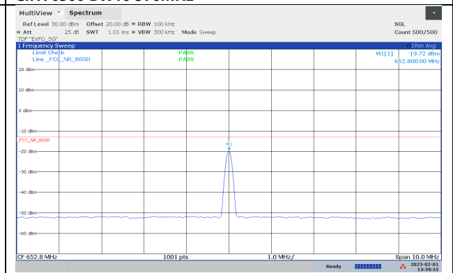
Ch176300 BW10 652.8MHz
