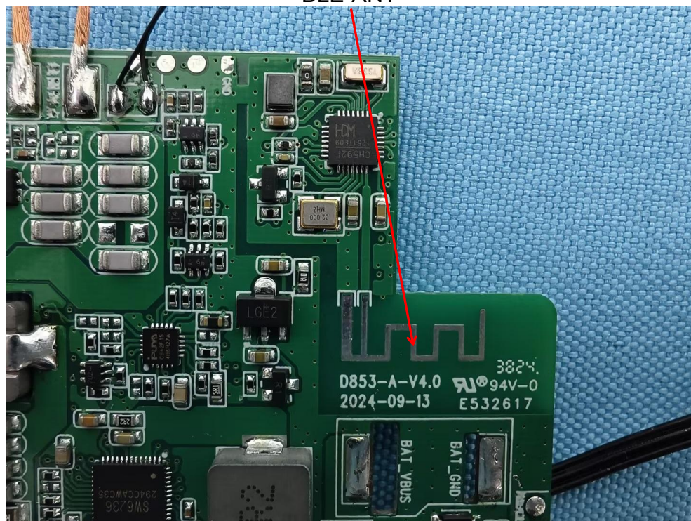
BLE-ANT
