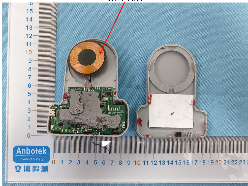
WPT-ANT
