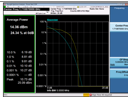
B4-3M-Low CH-PAPR-QPSK
