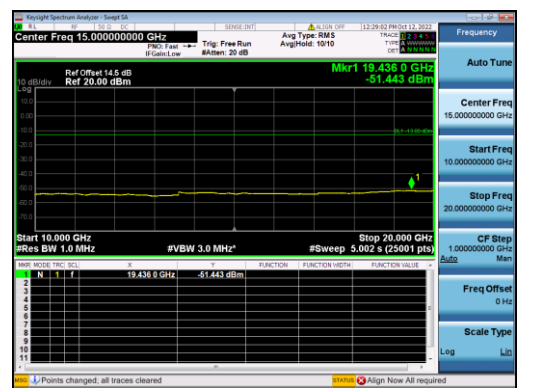
B4-10M-Low CH-CSE-2-Q16-1 RB 0
