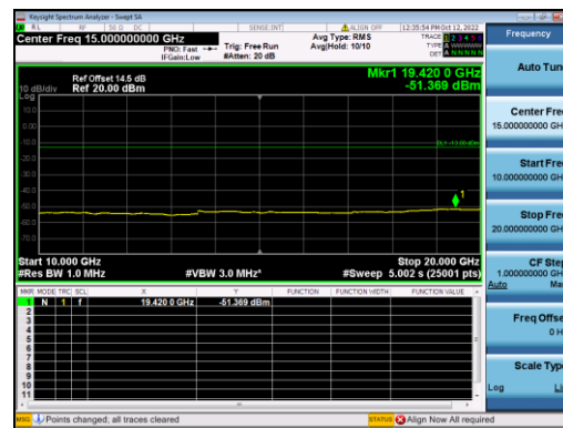
B4-15M-Low CH-CSE-2-Q16-1 RB 0
