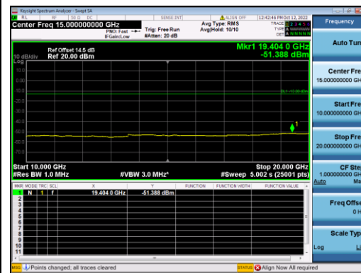
B4-20M-Low CH-CSE-2-Q16-1 RB 0
