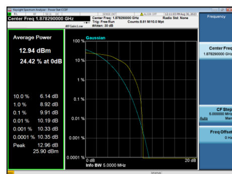
B2-5M-Mid CH-PAPR-Q16
