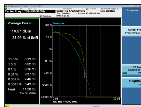
B4-15M-Mid CH-PAPR-QPSK
