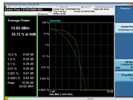
B2-15M-Mid CH-PAPR-QPSK
