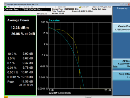
B4-10M-Mid CH-PAPR-QPSK
