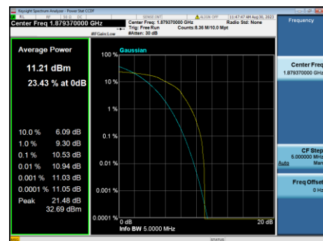
B2-3M-Mid CH-PAPR-Q16
