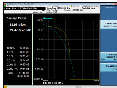
B2-20M-Mid CH-PAPR-Q16
