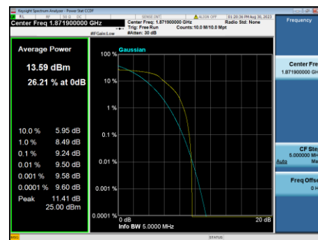
B2-20M-Mid CH-PAPR-QPSK
