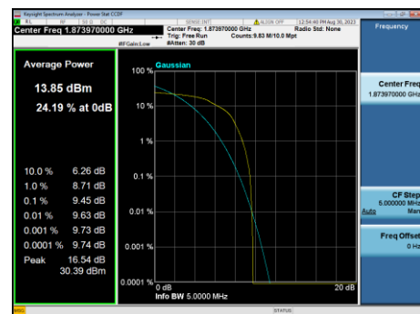
B2-15M-Mid CH-PAPR-Q16
