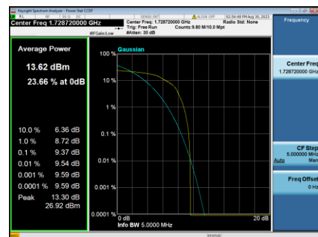
B4-10M-Mid CH-PAPR-Q16
