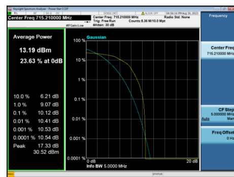
B12-5M-Low CH-PAPR-Q16
