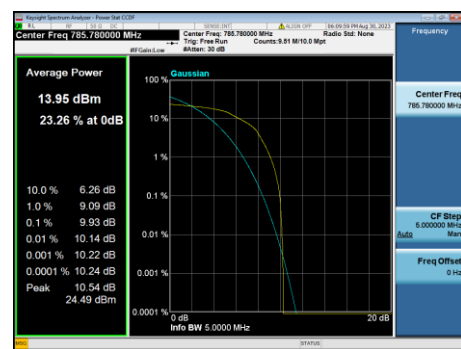
B13-10M-Low CH-PAPR-Q16
