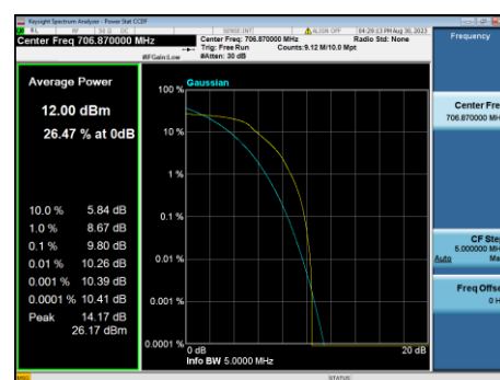
B12-3M-Mid CH-PAPR-QPSK
