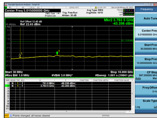
B13-10M-Mid CH-CSE-1-Q16-1 RB 0
