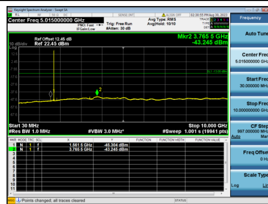
B4-5M-Mid CH-CSE-1-Q16-1 RB 0
