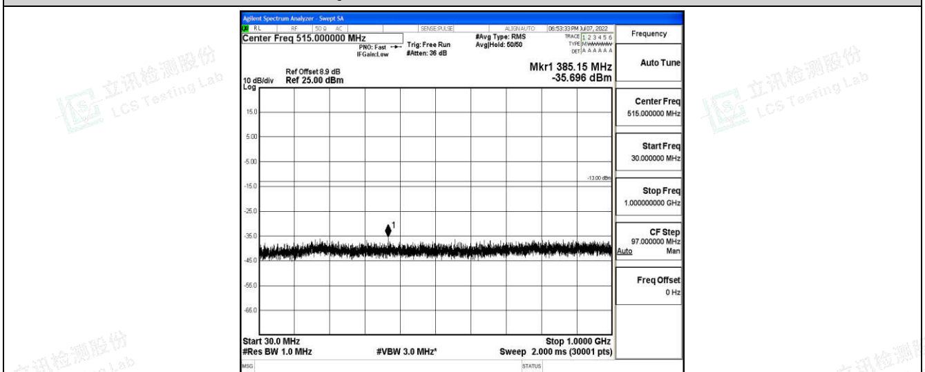
Band2-5MHz-16QAM-18900-1-0-Low-30-1000--35.7-PASS
