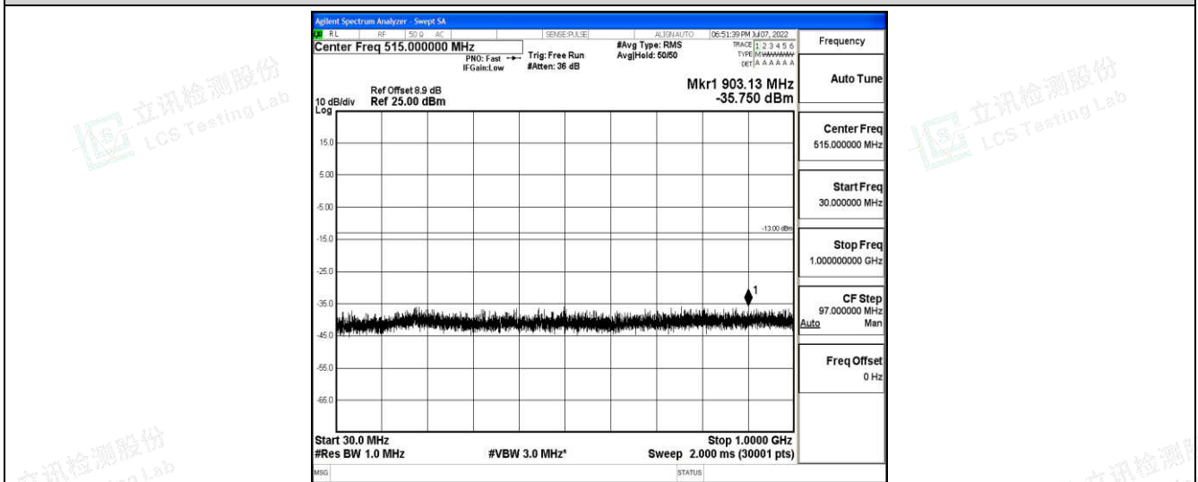
Band2-5MHz-QPSK-18900-1-0-Low-30-1000--35.75-PASS
