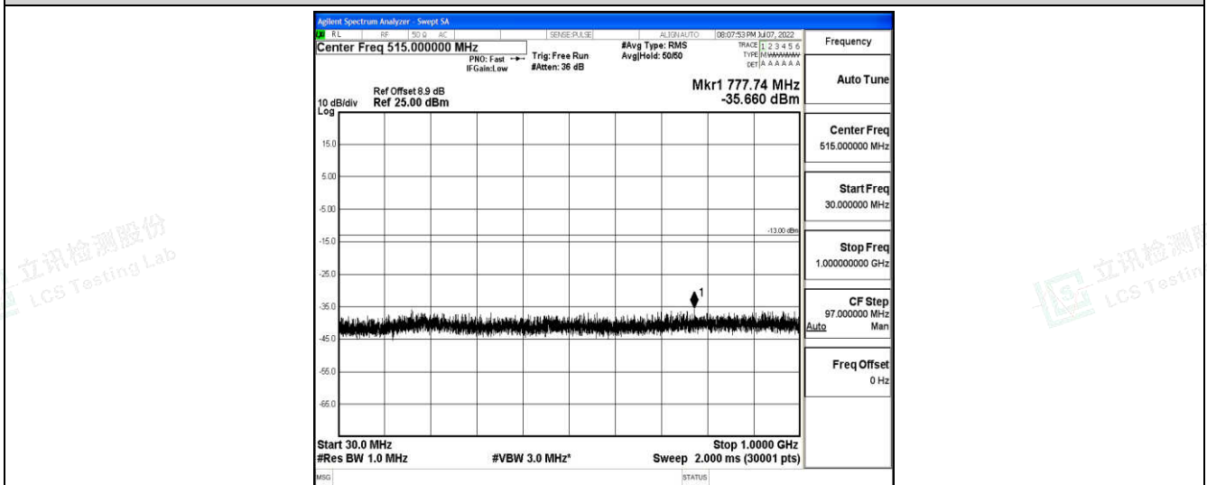
Band2-20MHz-16QAM-18700-1-0-Low-30-1000--35.66-PASS
