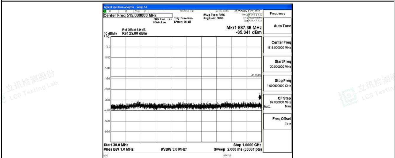
Band2-20MHz-QPSK-18700-1-0-Low-30-1000--35.34-PASS
