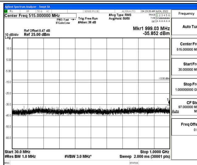
Band4-3MHz-QPSK-20175-1-0-Low-30-1000--35.85-PASS
