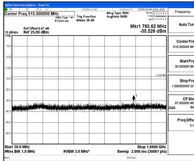
Band4-1.4MHz-QPSK-19957-1-0-Low-30-1000--35.53-PASS
