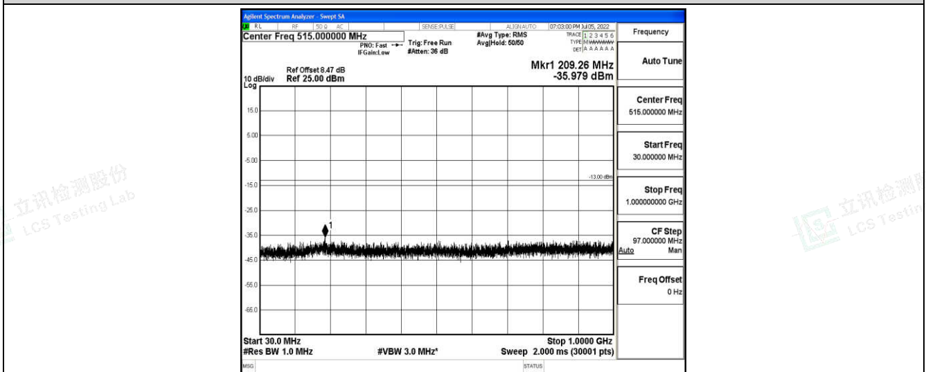
Band4-20MHz-QPSK-20050-1-0-Low-30-1000--35.98-PASS
