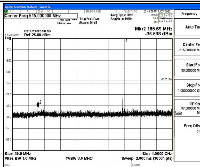
Band12-3MHz-QPSK-23095-1-0-Low-30-1000--36.7-PASS
