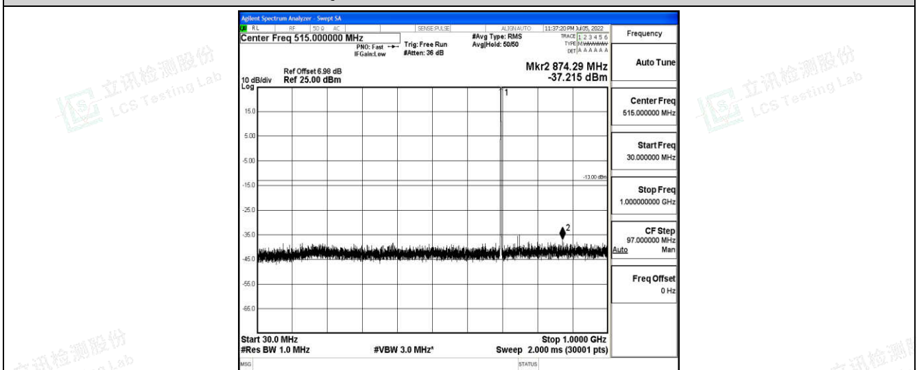
Band12-10MHz-QPSK-23095-1-0-Low-30-1000--37.22-PASS
