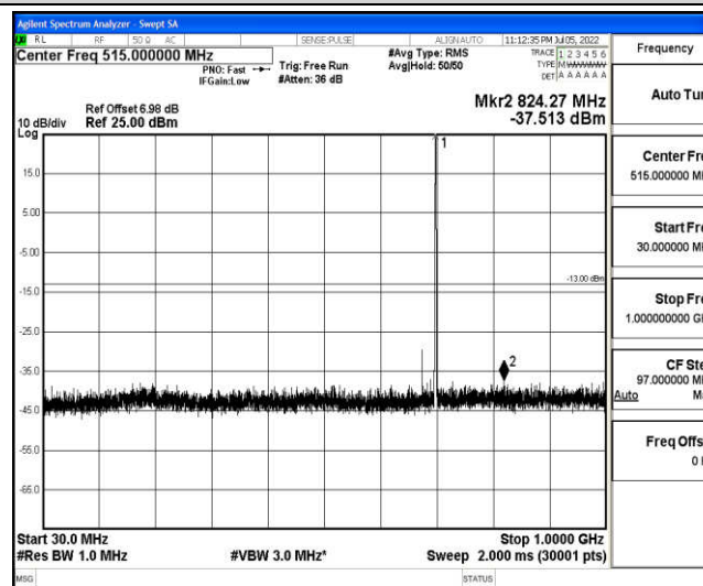
Band12-5MHz-16QAM-23095-1-0-Low-30-1000--37.51-PASS
