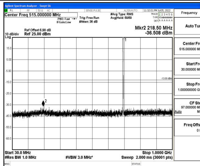
Band12-10MHz-QPSK-23060-1-0-Low-30-1000--36.51-PASS
