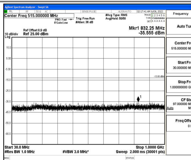
Band25-10MHz-QPSK-26365-1-0-Low-30-1000--35.56-PASS
