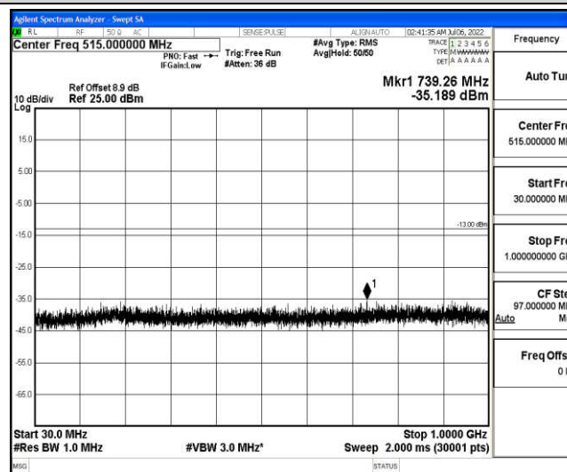
Band25-15MHz-QPSK-26365-1-0-Low-30-1000--35.19-PASS
