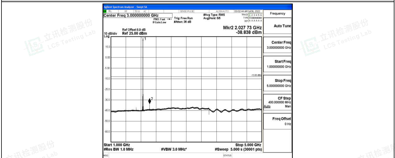
Band25-20MHz-QPSK-26140-1-0-Low-1000-5000--38.84-PASS
