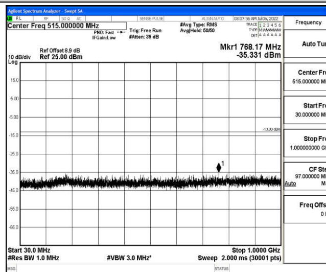
Band25-20MHz-16QAM-26365-1-0-Low-30-1000--35.33-PASS
