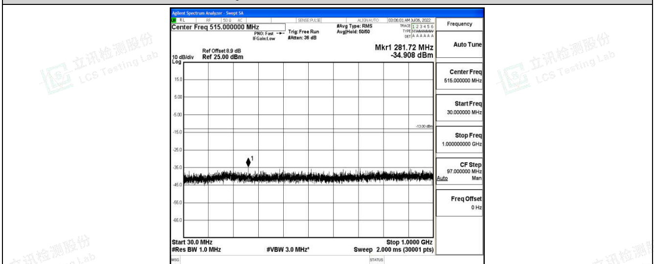
Band25-20MHz-QPSK-26365-1-0-Low-30-1000--34.91-PASS
