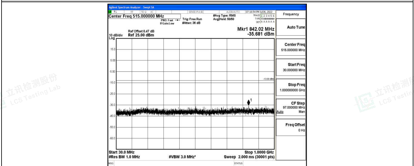
Band66-10MHz-QPSK-132022-1-0-Low-30-1000--35.68-PASS
