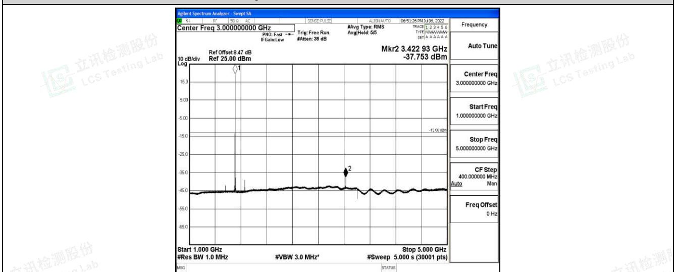
Band66-20MHz-QPSK-132072-1-0-Low-1000-5000--37.75-PASS
