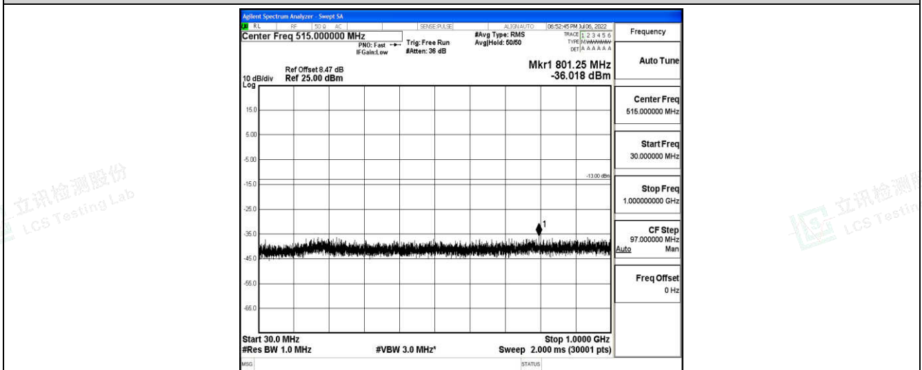
Band66-20MHz-16QAM-132072-1-0-Low-30-1000--36.02-PASS
