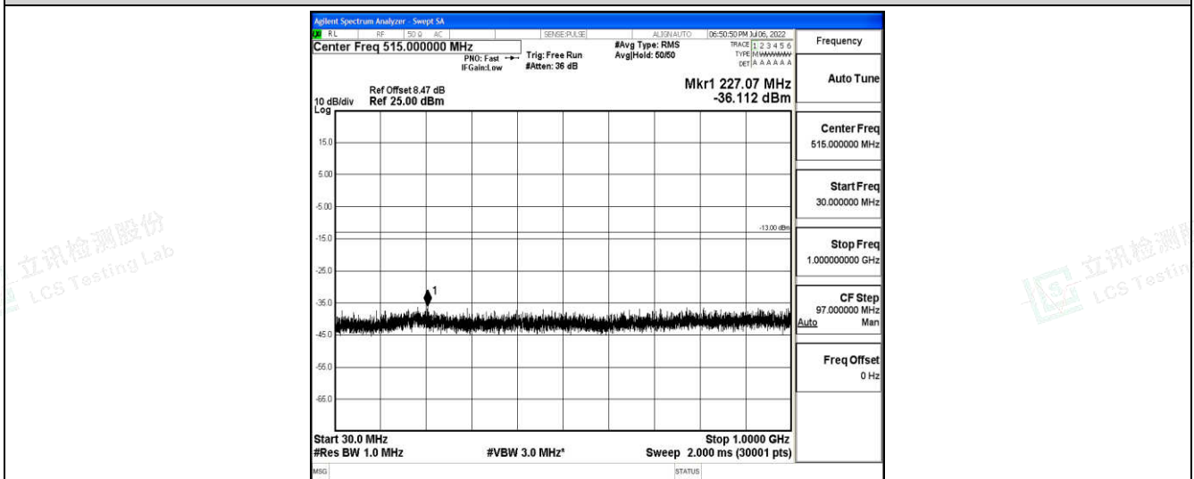
Band66-20MHz-QPSK-132072-1-0-Low-30-1000--36.11-PASS
