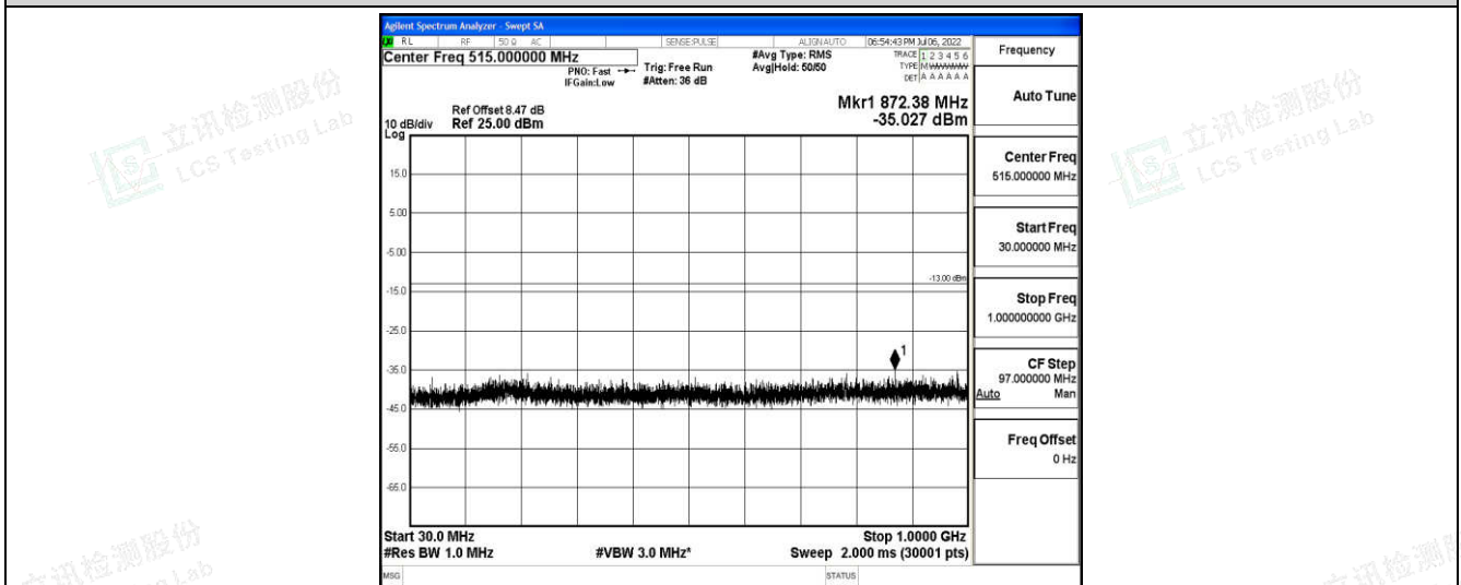
Band66-20MHz-QPSK-132322-1-0-Low-30-1000--35.03-PASS
