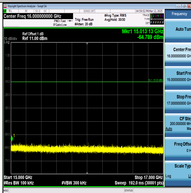
BLE_2M-Ant1-2402-15000~17000-PASS
