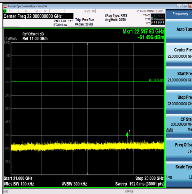
BLE_2M-Ant1-2440-21000~23000-PASS
