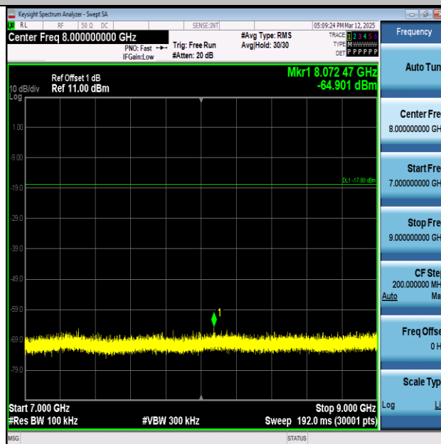
BLE_2M-Ant1-2480-7000~9000-PASS
