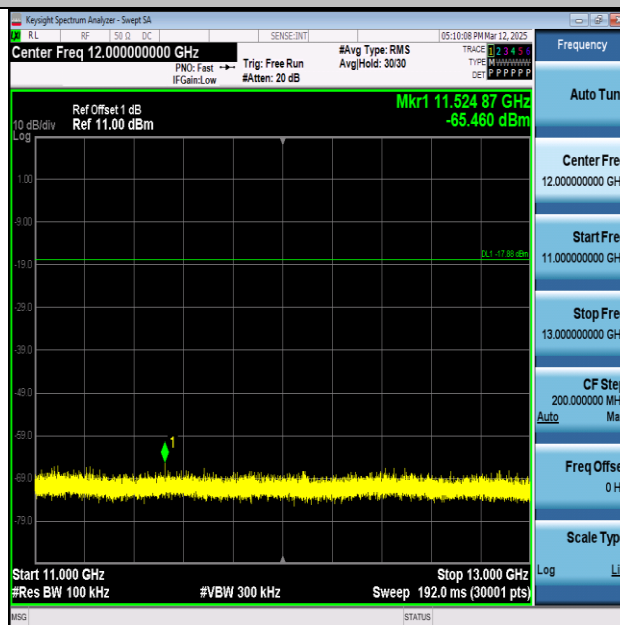
BLE_2M-Ant1-2480-11000~13000-PASS
