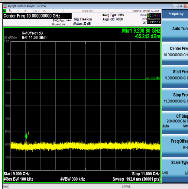
BLE_2M-Ant1-2440-9000~11000-PASS
