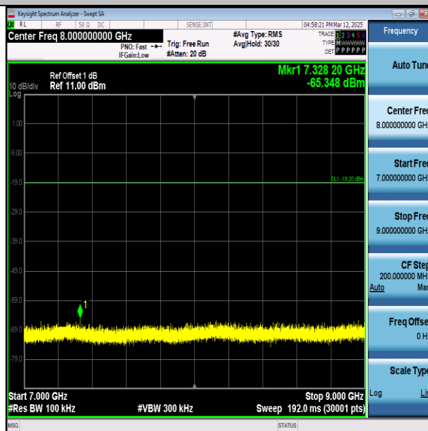
BLE_2M-Ant1-2402-7000~9000-PASS
