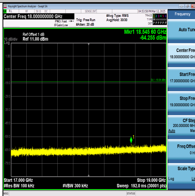
BLE_1M-Ant1-2480-17000~19000-PASS
