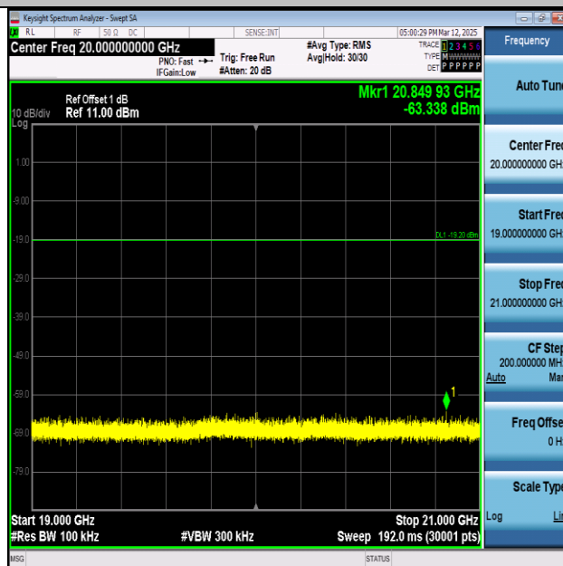
BLE_2M-Ant1-2402-19000~21000-PASS
