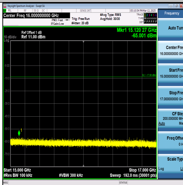
BLE_2M-Ant1-2480-15000~17000-PASS
