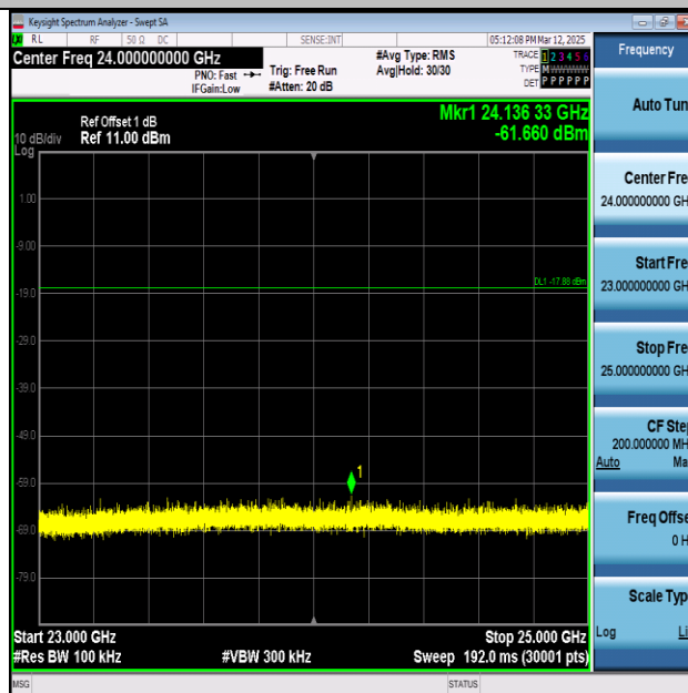
BLE_2M-Ant1-2480-23000~25000-PASS
