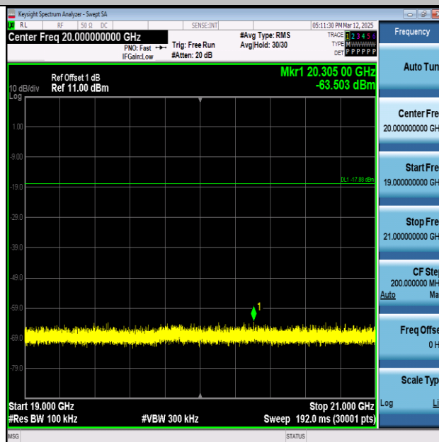
BLE_2M-Ant1-2480-19000~21000-PASS
