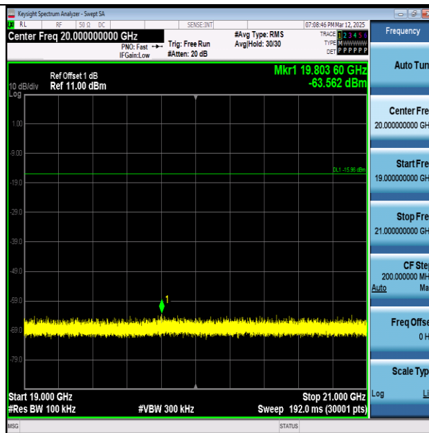
DH5-Ant1-2480-19000~21000-PASS
