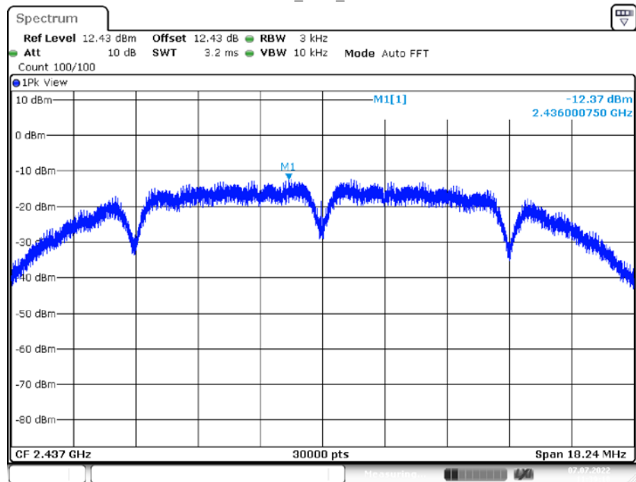
11B_Ant1_2437
