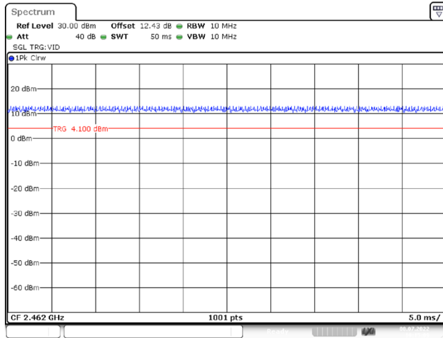
11G_Ant1_2462
