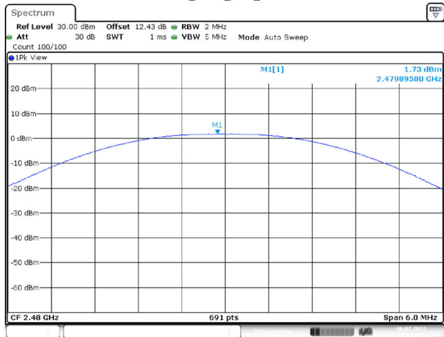
BLE_BT4.0_Ant1_2480
