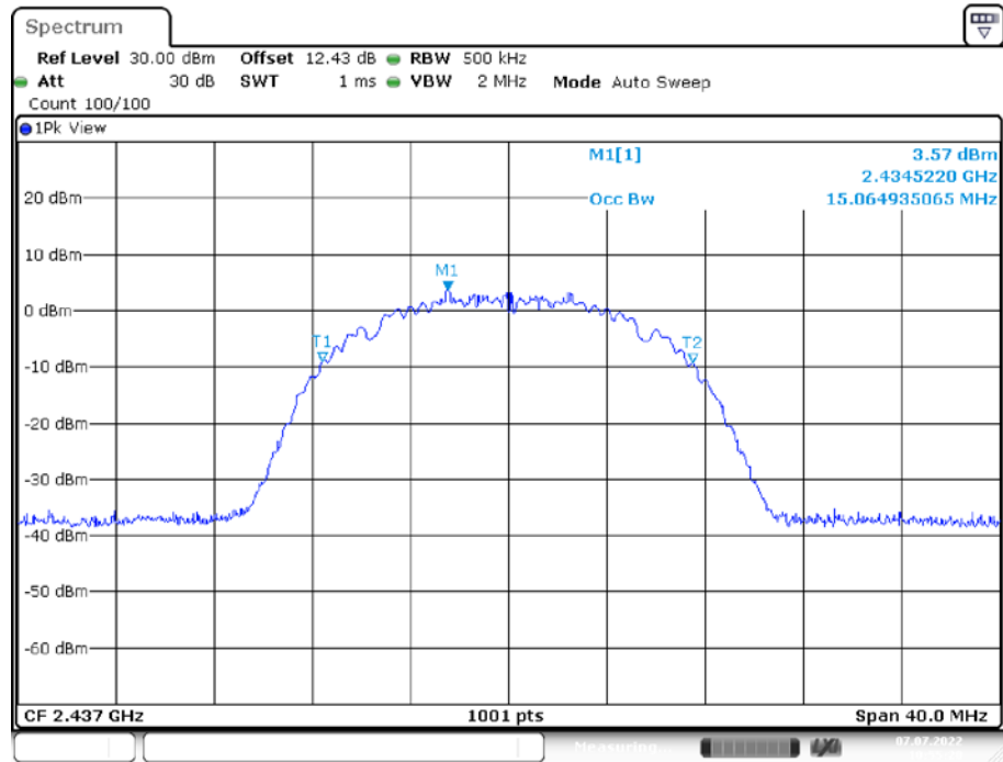
11B_Ant1_2437
