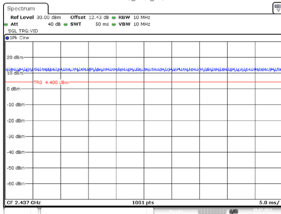
11G_Ant1_2437
