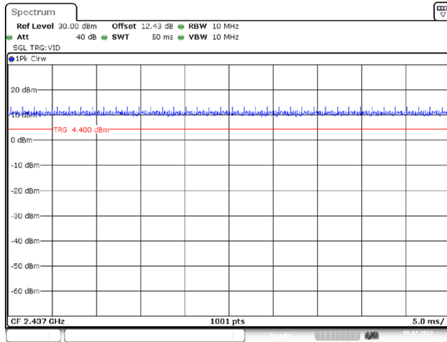
11N20SISO_Ant1_2437
