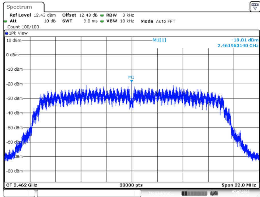
11G_Ant1_2462
