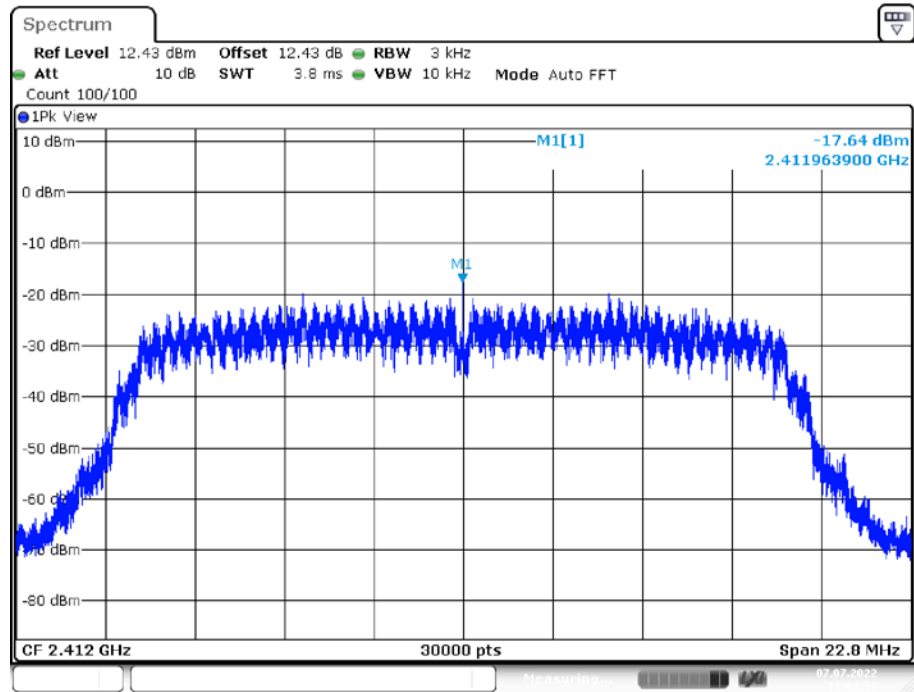
11G_Ant1_2412
