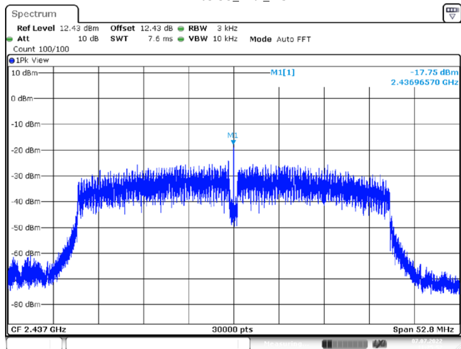
11N40SISO_Ant1_2437
