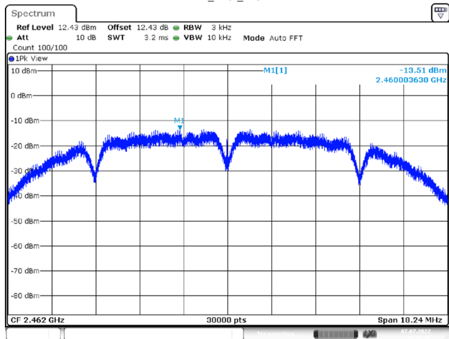
11B_Ant1_2462
