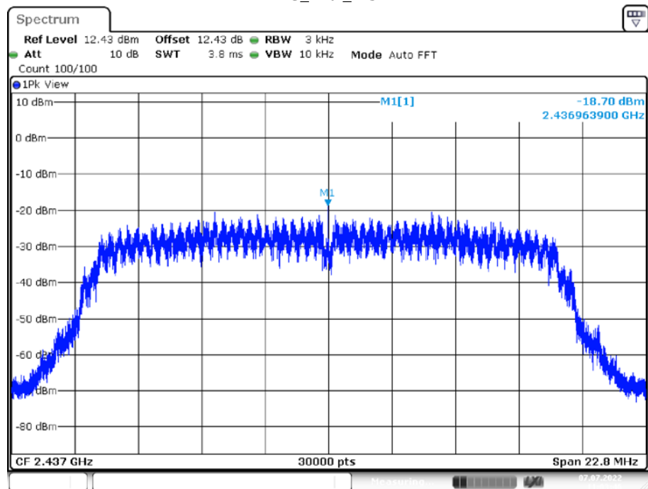
11G_Ant1_2437
