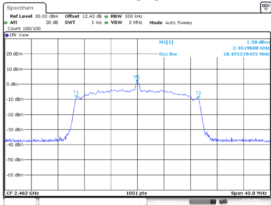
11N20SISO_Ant1_2462
