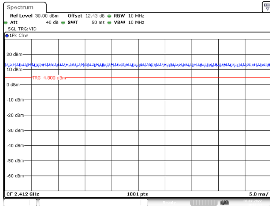
11G_Ant1_2412
