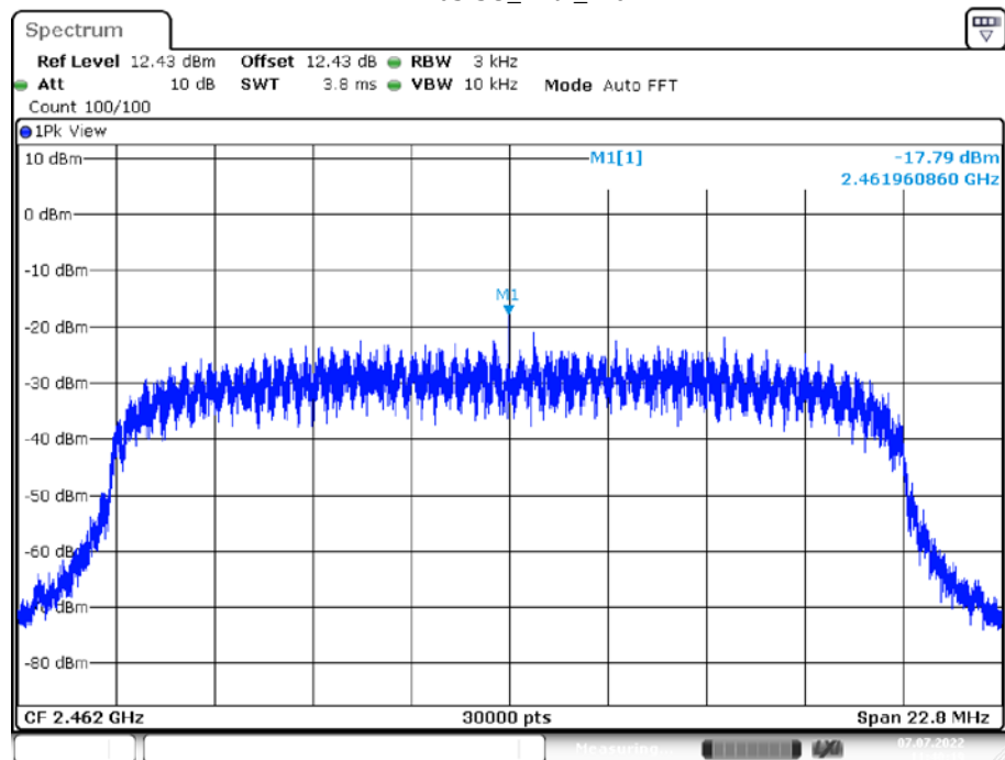
11N20SISO_Ant1_2462
