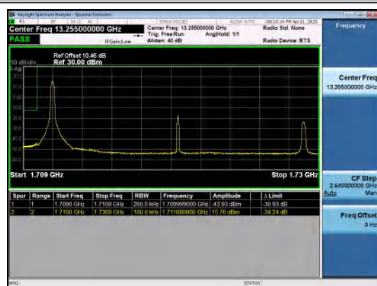
Band4-20MHz-QPSK-20050-1RB#0-PASS
