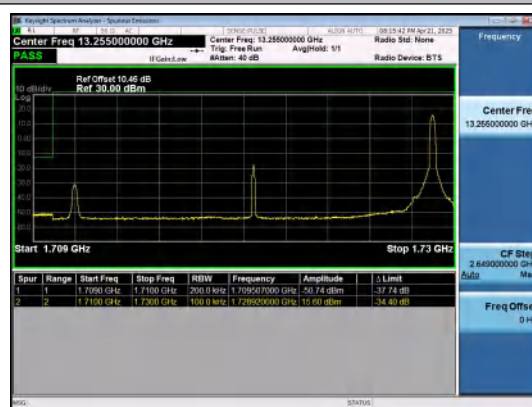
Band4-20MHz-QPSK-20050-1RB#99-PASS
