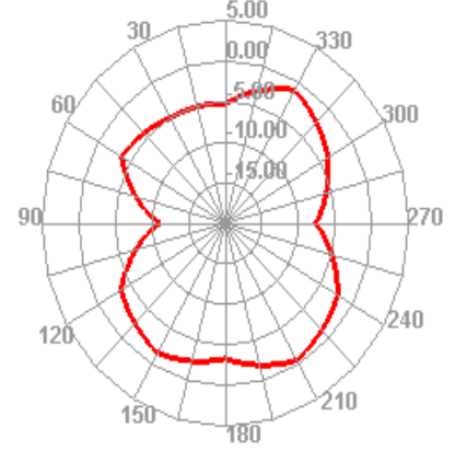
2410.000MHz E2
