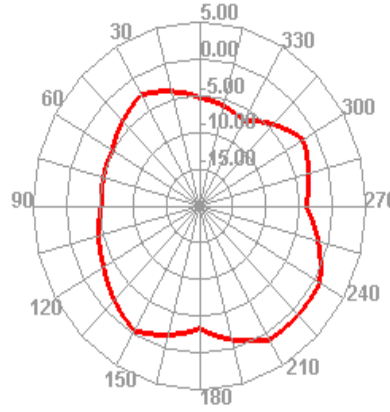
2410.000MHz E1
