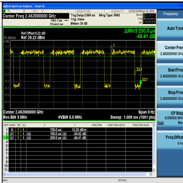
NTNV-11N20MIMO-Ant1-2462
