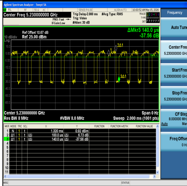
NTNV-11AC40MIMO-Ant1-5230
