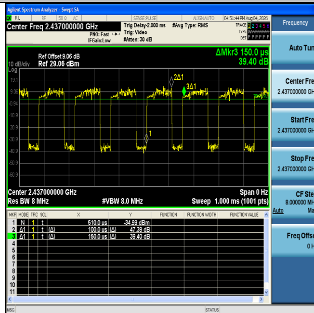
NTNV-11N40MIMO-Ant2-2437
