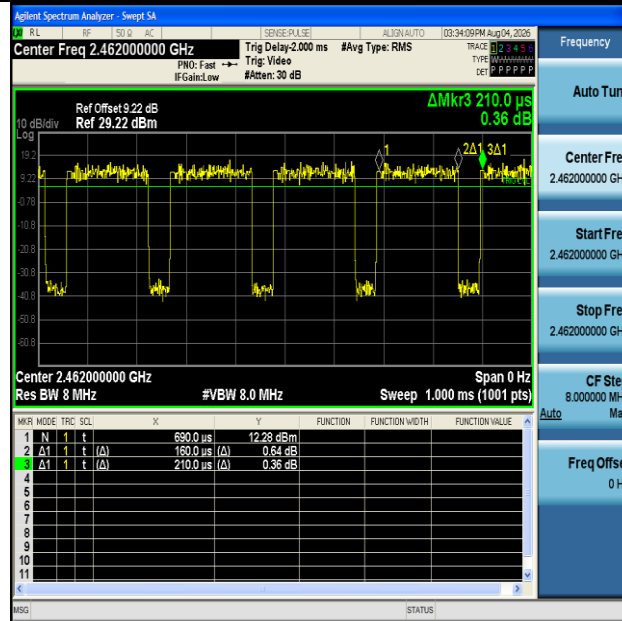
NTNV-11N20MIMO-Ant1-2462
