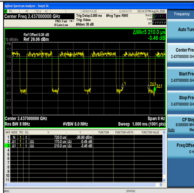
NTNV-11N20MIMO-Ant2-2437
