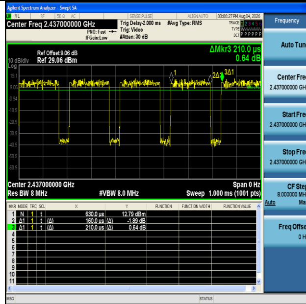
NTNV-11N20MIMO-Ant1-2437
