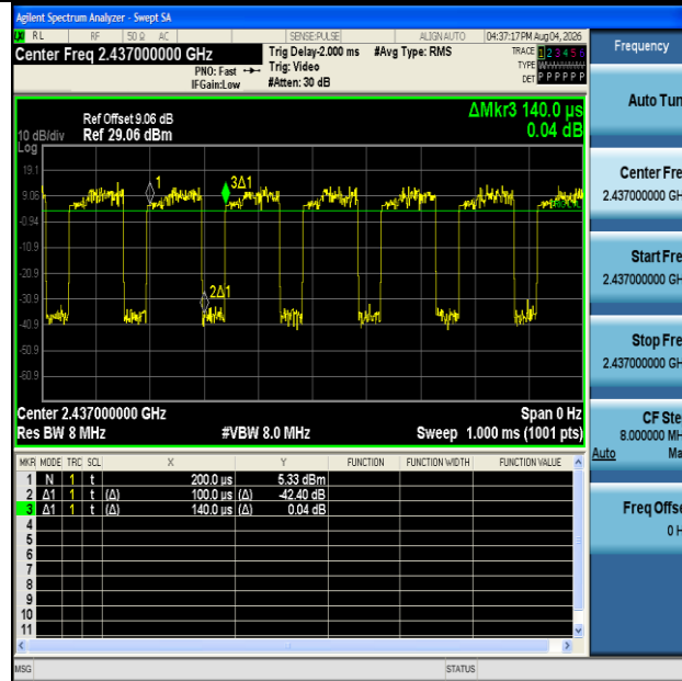
NTNV-11N40MIMO-Ant1-2437
