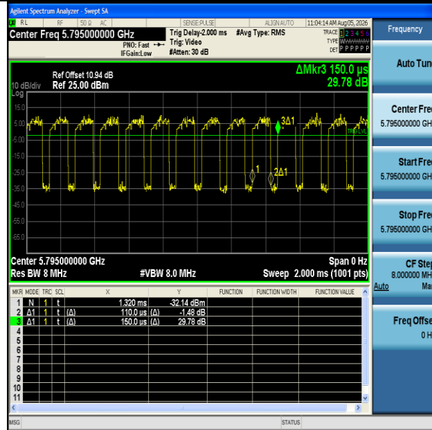
NTNV-11AC40MIMO-Ant1-5795
