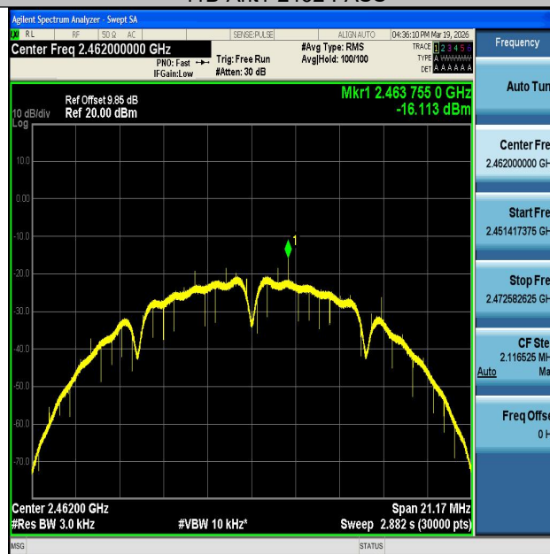
11B-Ant2-2462-PASS
