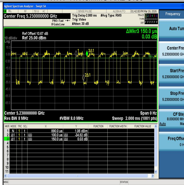
NTNV-11N40MIMO-Ant1-5230
