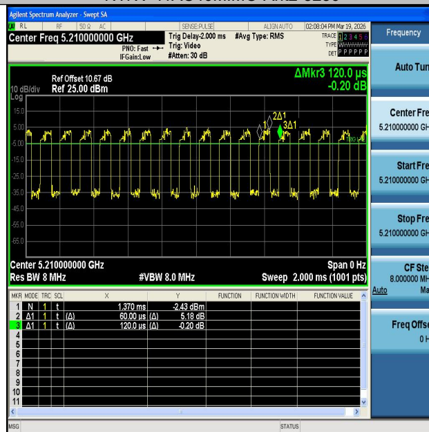
NTNV-11AC80MIMO-Ant1-5210
