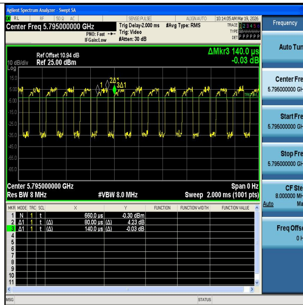
NTNV-11AC40MIMO-Ant1-5795
