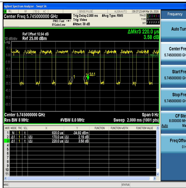
NTNV-11N20MIMO-Ant1-5745
