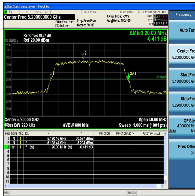
11AC20MIMO-Ant1-5200
