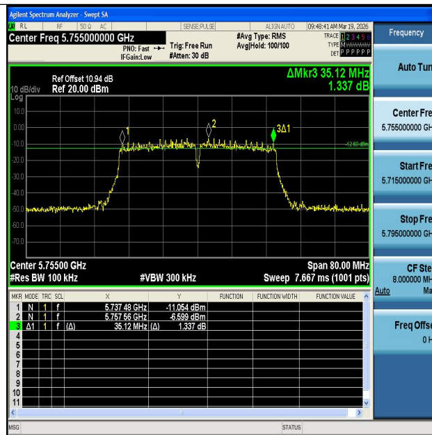
11N40MIMO-Ant1-5755-PASS
