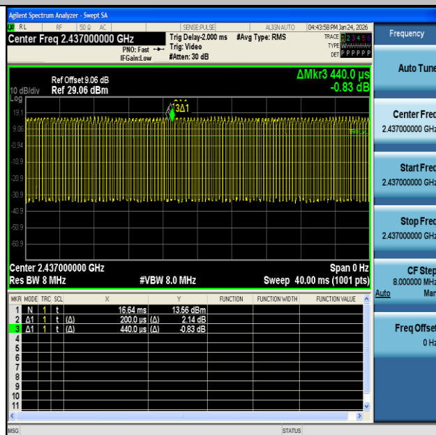
NTNV-11N20MIMO-Ant2-2437
