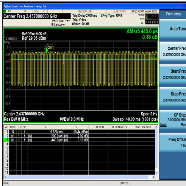
NTNV-11N20MIMO-Ant1-2437
