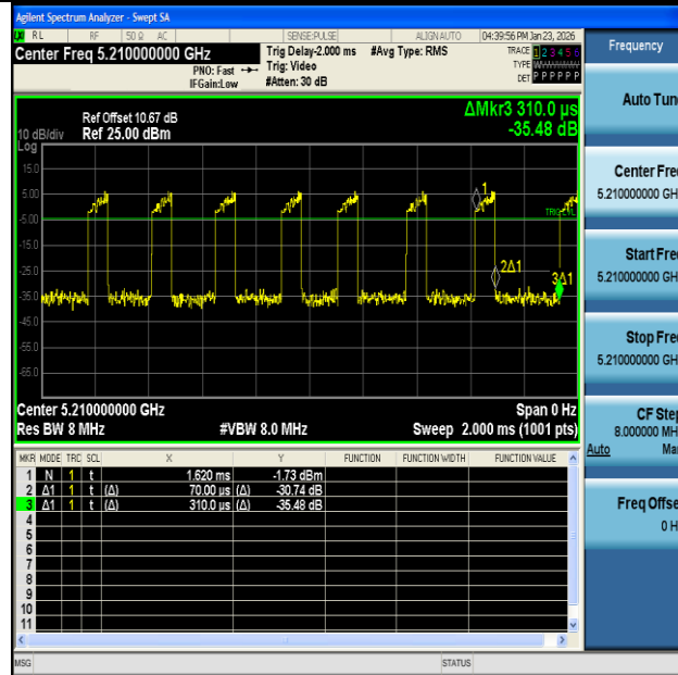
NTNV-11AC80MIMO-Ant1-5210
