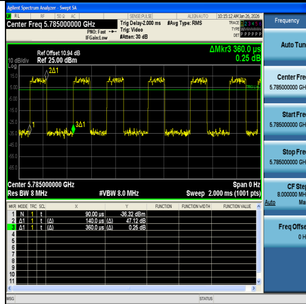
NTNV-11N20MIMO-Ant1-5785
