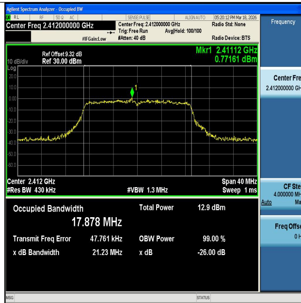
11N20MIMO-Ant1-2412
