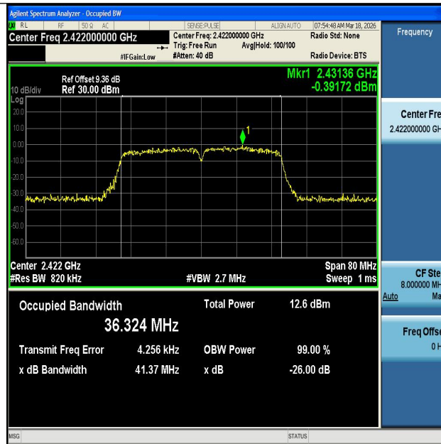
11N40MIMO-Ant1-2422
