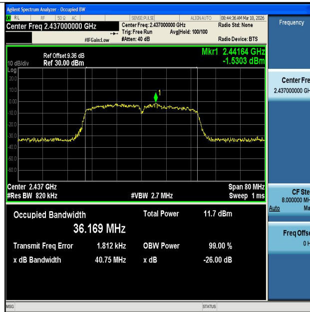
11N40MIMO-Ant1-2437
