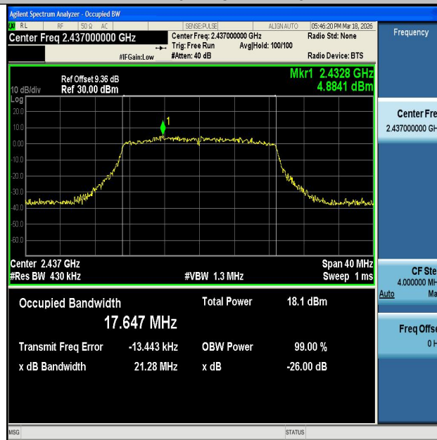
11N20MIMO-Ant2-2437
