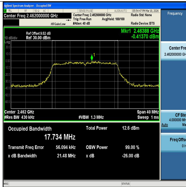
11N20MIMO-Ant1-2462
