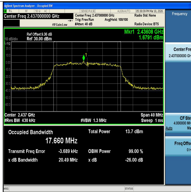
11N20MIMO-Ant1-2437
