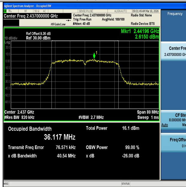
11N40MIMO-Ant2-2437
