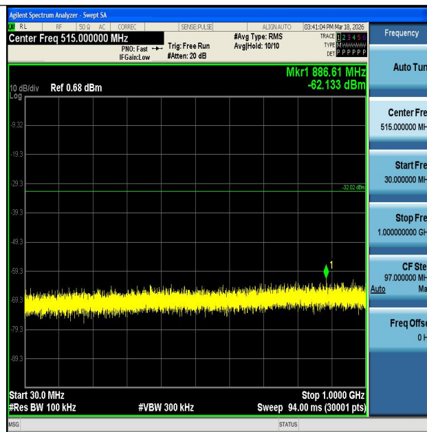
11G-Ant1-2412-30~1000-PASS
