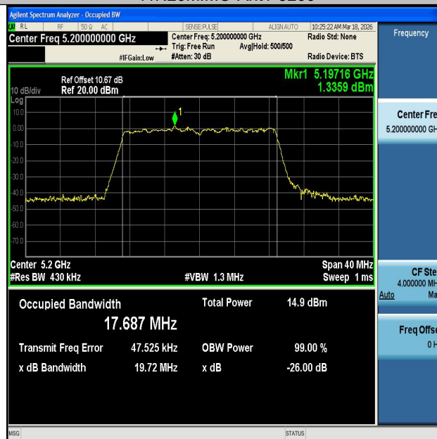
11N20MIMO-Ant2-5200
