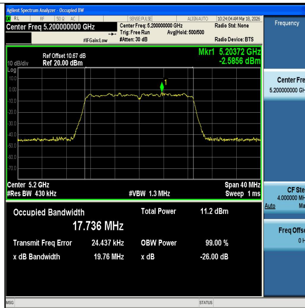
11N20MIMO-Ant1-5200
