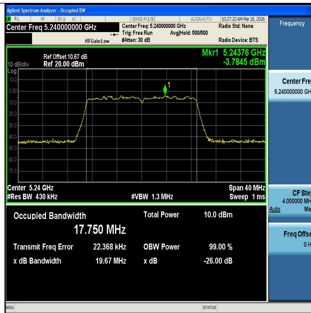
11N20MIMO-Ant1-5240
