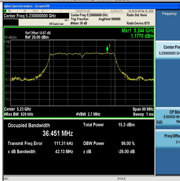
11N40MIMO-Ant2-5230
