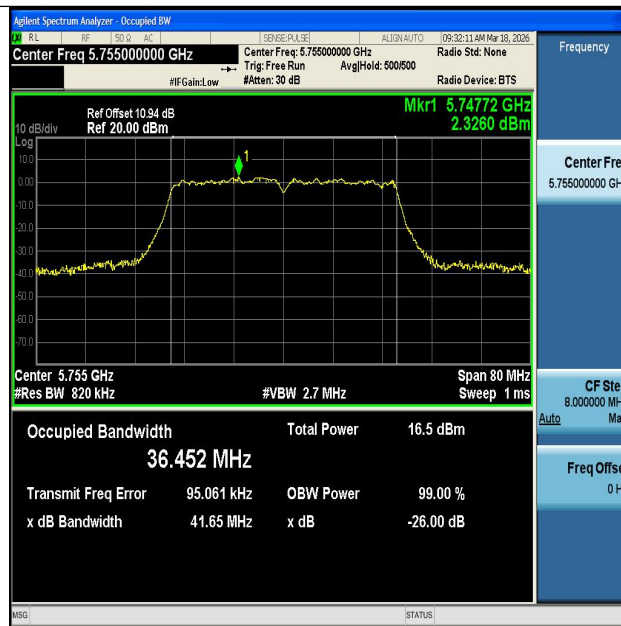
11N40MIMO-Ant1-5755
