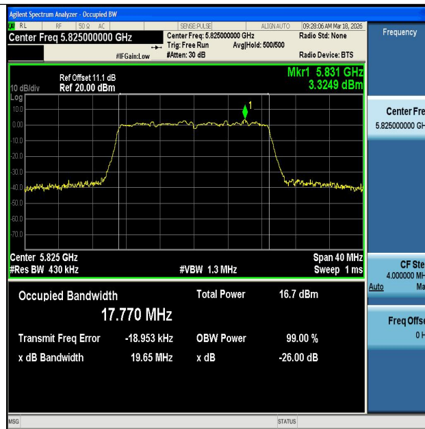
11N20MIMO-Ant1-5825
