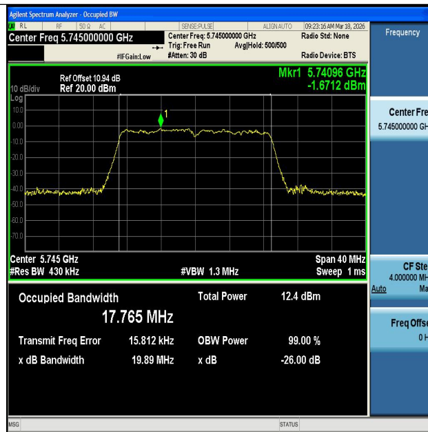
11N20MIMO-Ant1-5745
