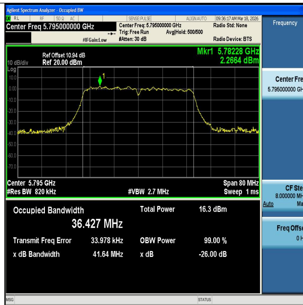
11N40MIMO-Ant1-5795
