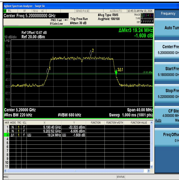
11AC20MIMO-Ant1-5200
