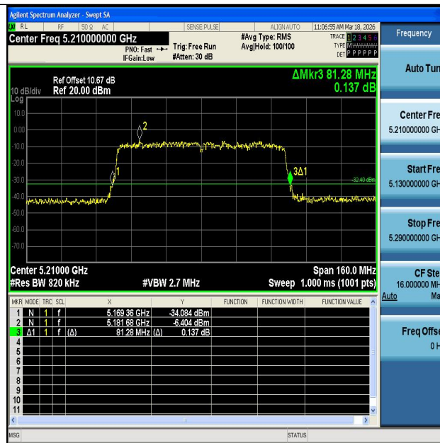
11AC80MIMO-Ant1-5210
