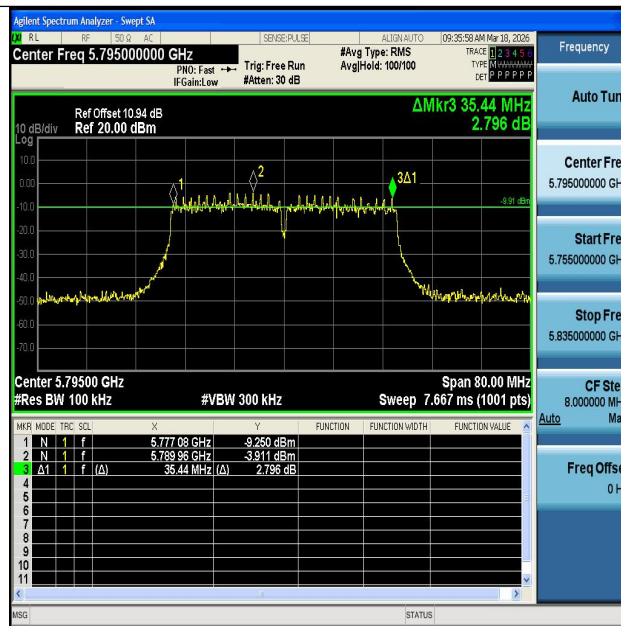
11N40MIMO-Ant1-5795-PASS
