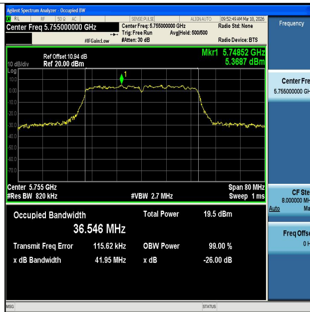
11AC40MIMO-Ant1-5755
