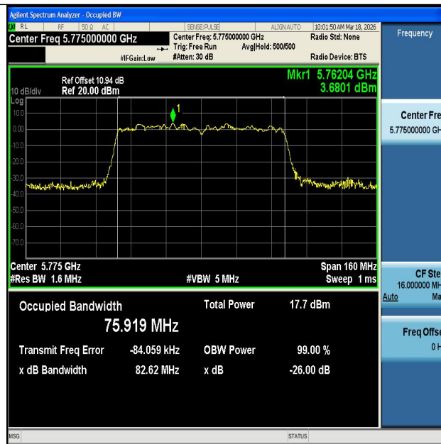
11AC80MIMO-Ant1-5775
