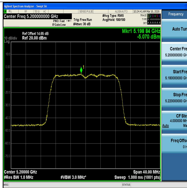
11N20MIMO-Ant1-5200-PASS
