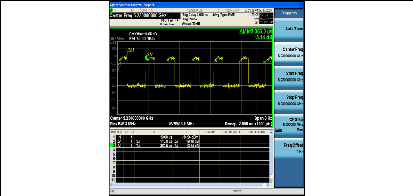
NTNV-11AC40MIMO-Ant1-5230
