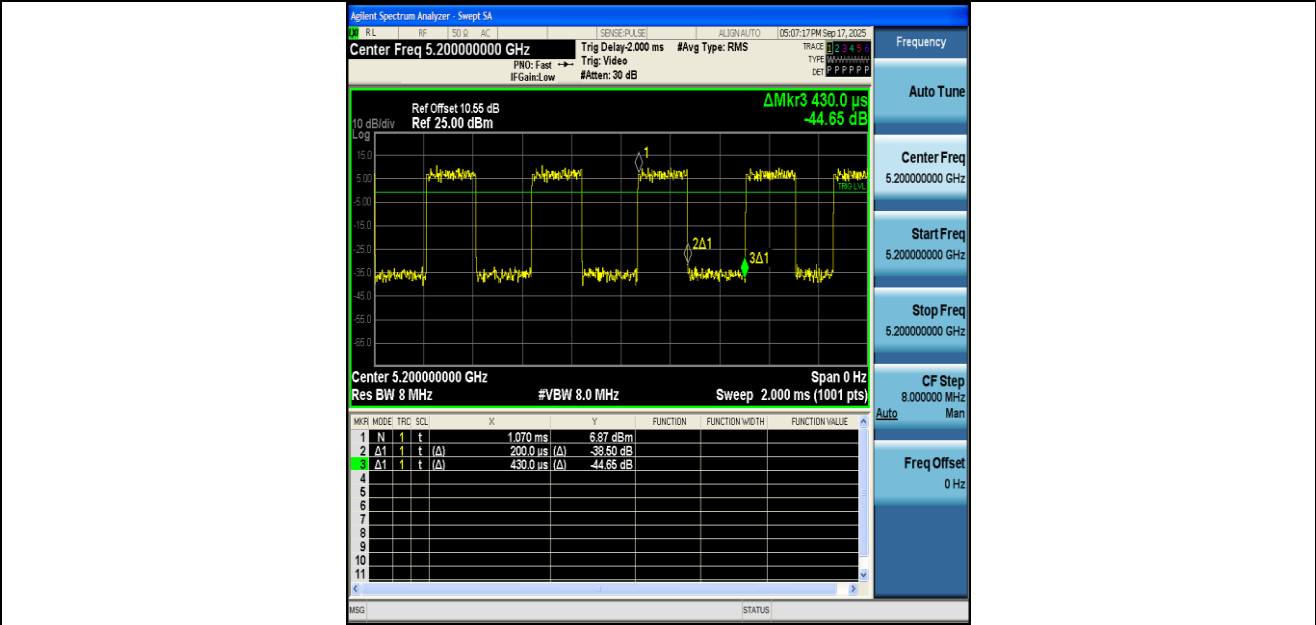
NTNV-11AC20MIMO-Ant1-5200
