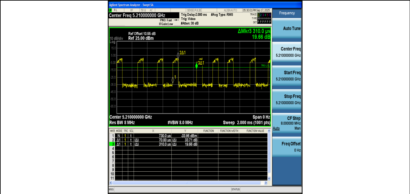
NTNV-11AC80MIMO-Ant1-5210
