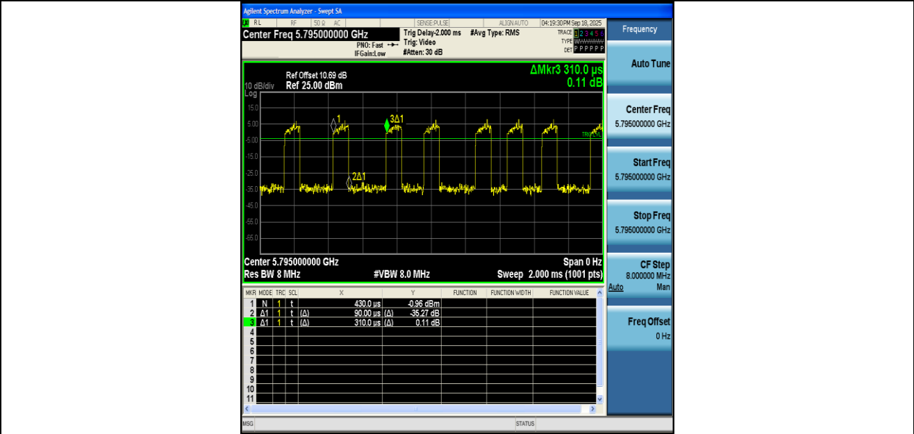
NTNV-11N40MIMO-Ant1-5795
