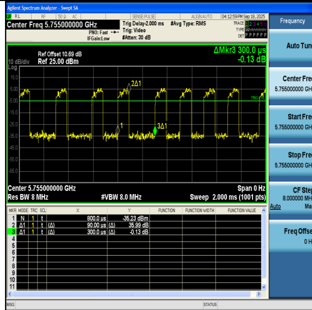
NTNV-11N40MIMO-Ant1-5755
