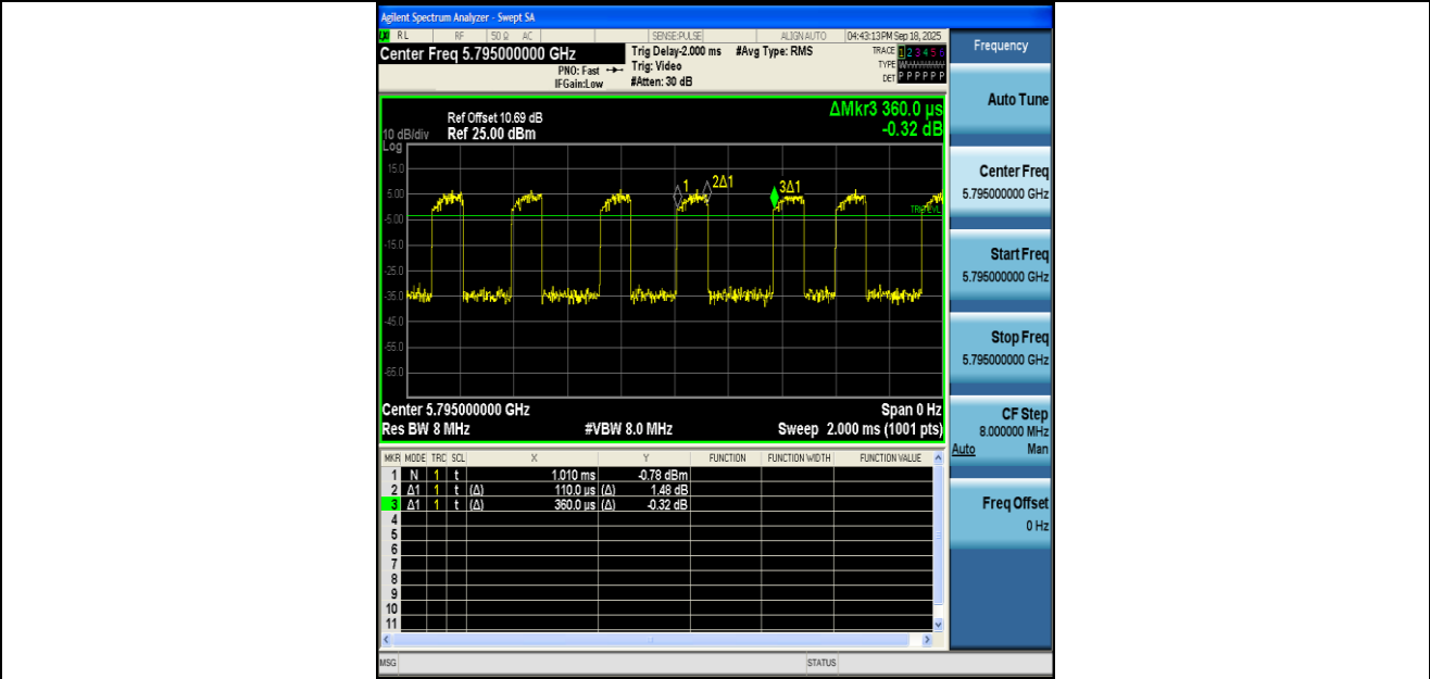
NTNV-11AC40MIMO-Ant1-5795
