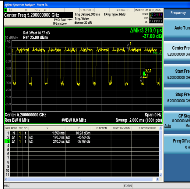
NTNV-11AC20MIMO-Ant1-5200
