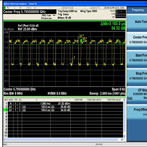
NTNV-11N40MIMO-Ant1-5795
