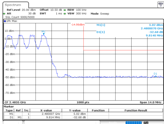
DH1_Hopping_Upper
