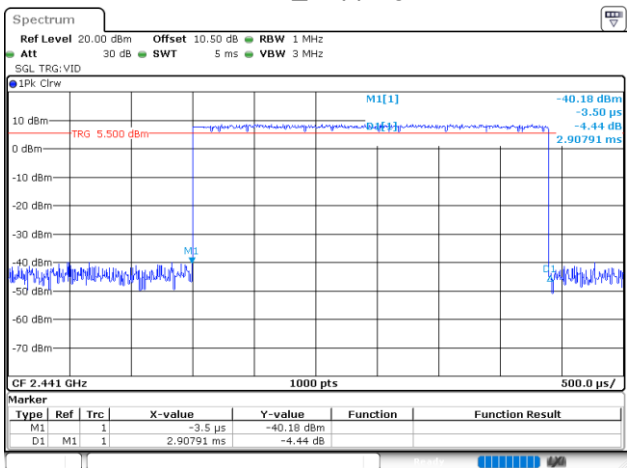
2DH5_Hopping
