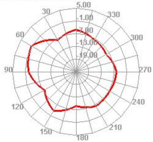
2400.000MHz H
