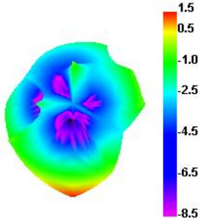
5150.000MHz
