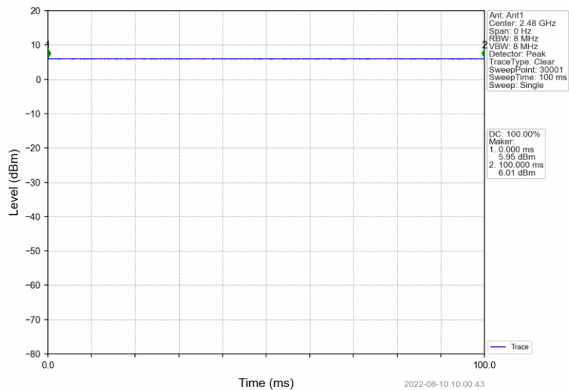
2M_HCH_2480MHz_Ant1_NTNV
