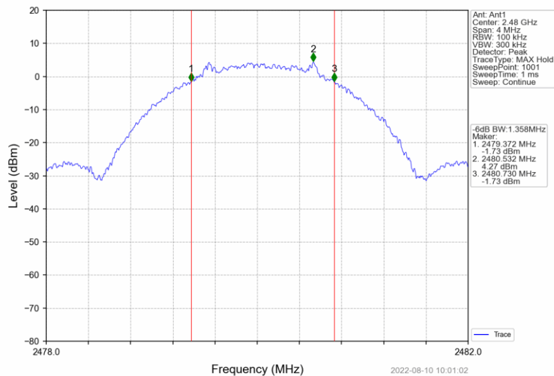
2M_HCH_2480MHz_Ant1_NTNV
